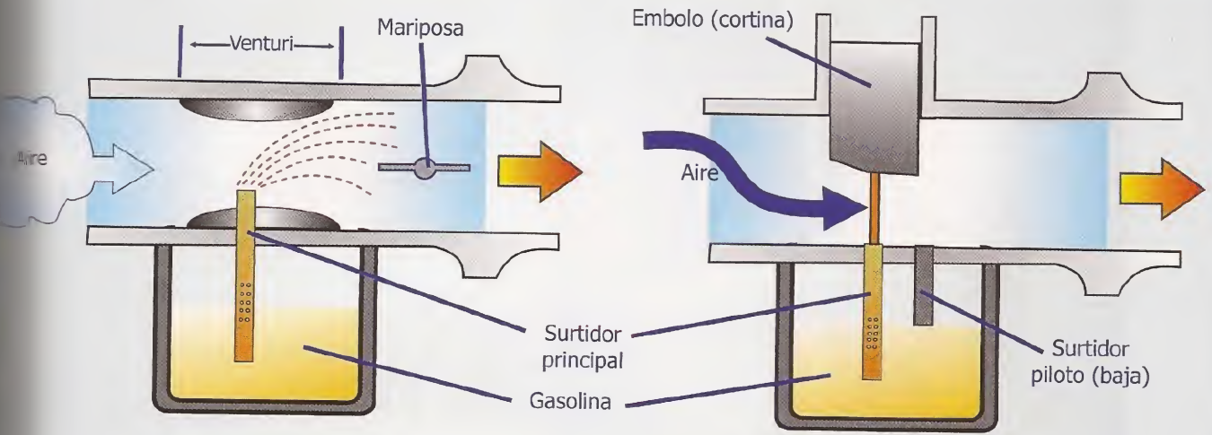
Principio venturi
